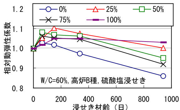
図－10 相対動弾性係数の経時変化
