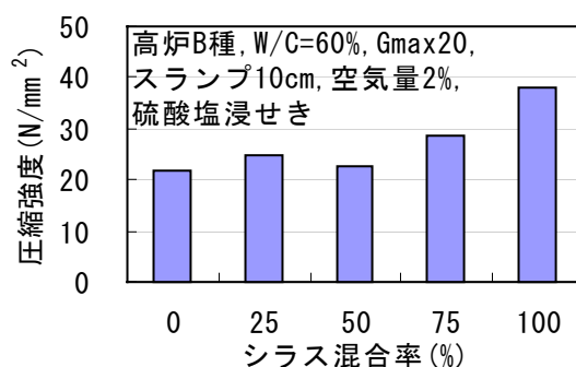
図-11 圧縮強度とシラス混合率の関係
