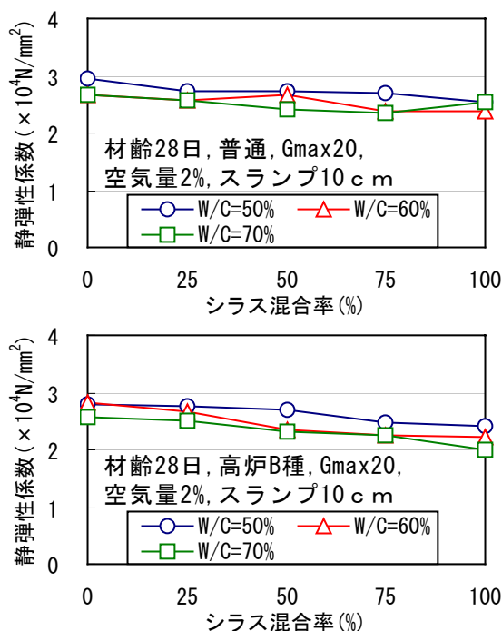
図－6 静弾性係数とシラス混合率の関係
