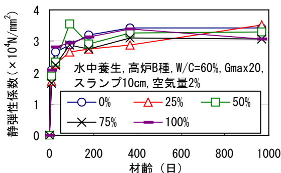
図－7 静弾性係数の経時変化
