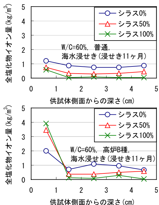
図-12 全塩化物イオン量分布
