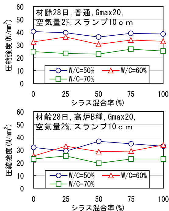
図-3 圧縮強度とシラス混合率の関係
