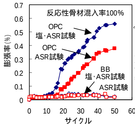
図 - 8 各試験のサイクル初期からの膨張率の経時変化
