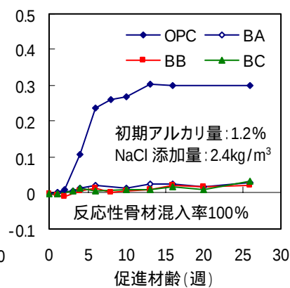
図 - 2 初期アルカリ量 1.2%の NaCl 添加量 2.4kg/m 3 における膨張率の経時変化
