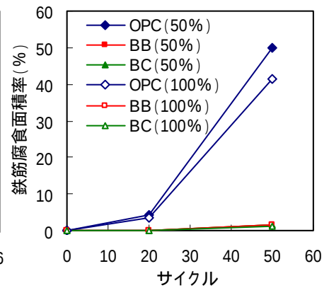
図 - 14 塩害 - ASR 試験の各供試体における鉄筋腐食面積率の経時変化
