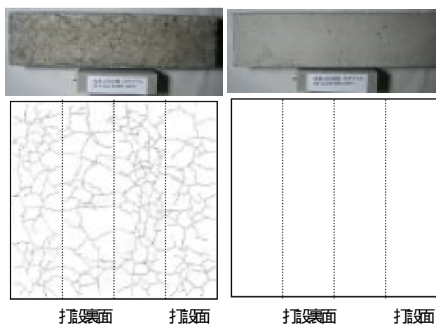
写真 - 1 塩害 - ASR 試験の 50 サイクル終了時の表面劣化写真および供試体ひび割れ状況
