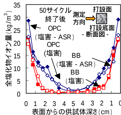
図 - 10 50 サイクル終了時の各試験の全塩化物イオン量分布
