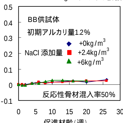
図 - 3 OPC および BB 供試体の反応性骨材混入率 50%における NaCl 添加量の違いによる膨張率の経時変化
