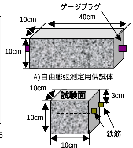
図 - 7 耐久性試験の供試体形状
