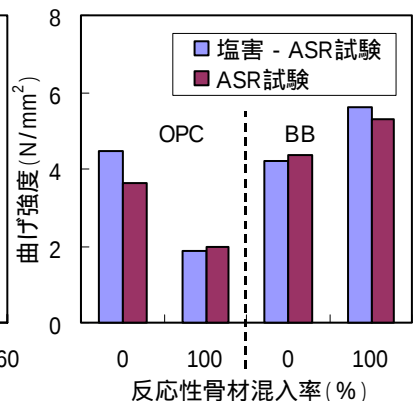
図 - 9 50 サイクル時の曲げ強度試験結果
