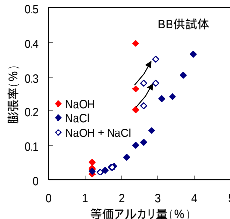
図 - 6 等価アルカリ量と膨張率の関係
