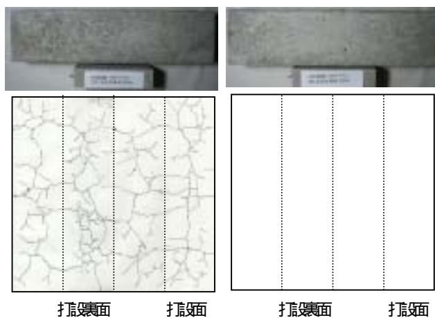
写真 - 2 ASR 試験の 50 サイクル終了時の表面劣化写真および供試体ひび割れ状況
