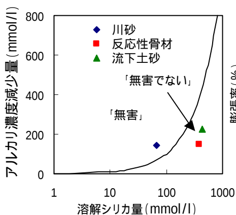
図 - 1 化学法結果
