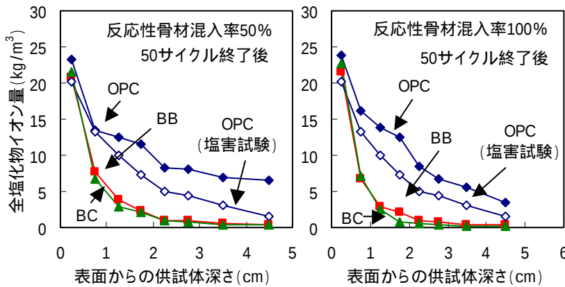
図 - 13 塩害 - ASR 試験あるいは塩害試験の 50 サイクル終了時における全塩化物イオン量分布
