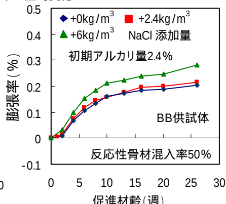
図 - 4 初期アルカリ量 2.4%の BB 供試体における膨張率の経時変化
