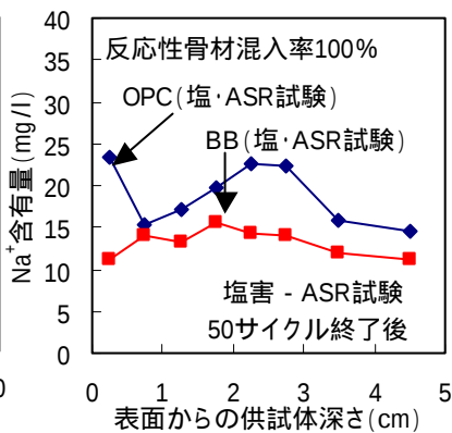
図 - 11 50 サイクル終了時の Na イオン含有量分布
