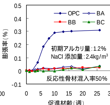
図 - 2 初期アルカリ量 1.2%の NaCl 添加量 2.4kg/m 3 における膨張率の経時変化
