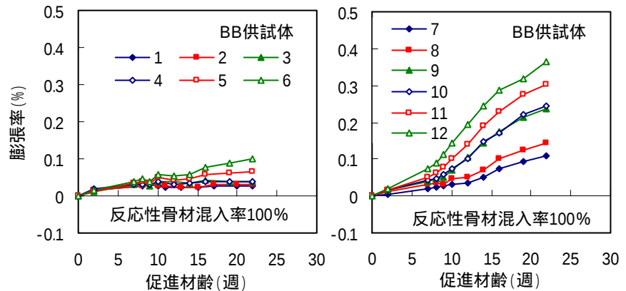
図 - 5 BB 供試体の反応性骨材混入率 100% における膨張率の経時変化
