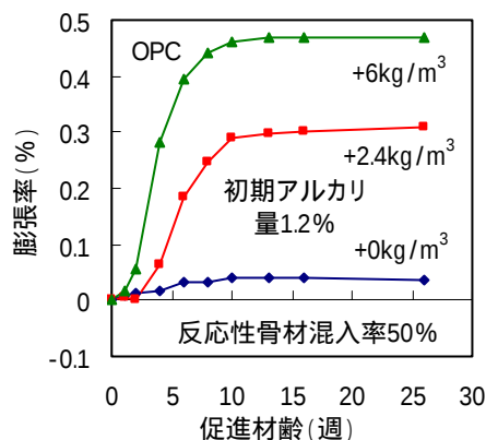
図 - 3 OPC および BB 供試体の反応性骨材混入率 50%における NaCl 添加量の違いによる膨張率の経時変化
