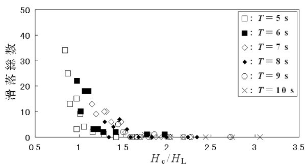
図-10 長周期波が入射する場合の消波ブロックの滑落総数（横軸は、天端高 H_c / 入射波波高 H_L である．）
