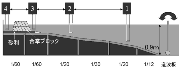
図-1 鉛直 2 次元造波水槽
