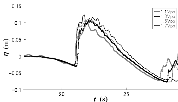
図-8 周期約 5.0 s の長周期波の堤前波形例
