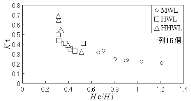
図-4 消波ブロックを 1 列に 16 個配置して組み上げた離岸堤に対する波高伝達率（ここで、各静水位の場合に対する波高伝達率 K_t = 堤背後波高 H_t / 堤前波高 H_i が示されている。横軸は、天端高 H_c / 堤前波高 H_i である。）
